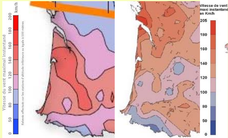
24 janvier 2009 et 27 décembre 1999 - Vitesse des vents Source Météo-France
